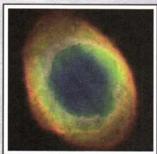
Рис. X. Планетарная туманность Кольцеобразная в созвездии Лиры.
