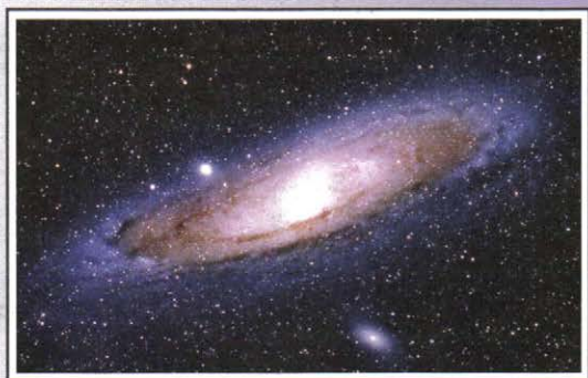
Рис. XIX. Туманность Андромеды.
