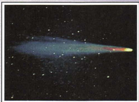
Рис. VIII. Комета Галлея.
